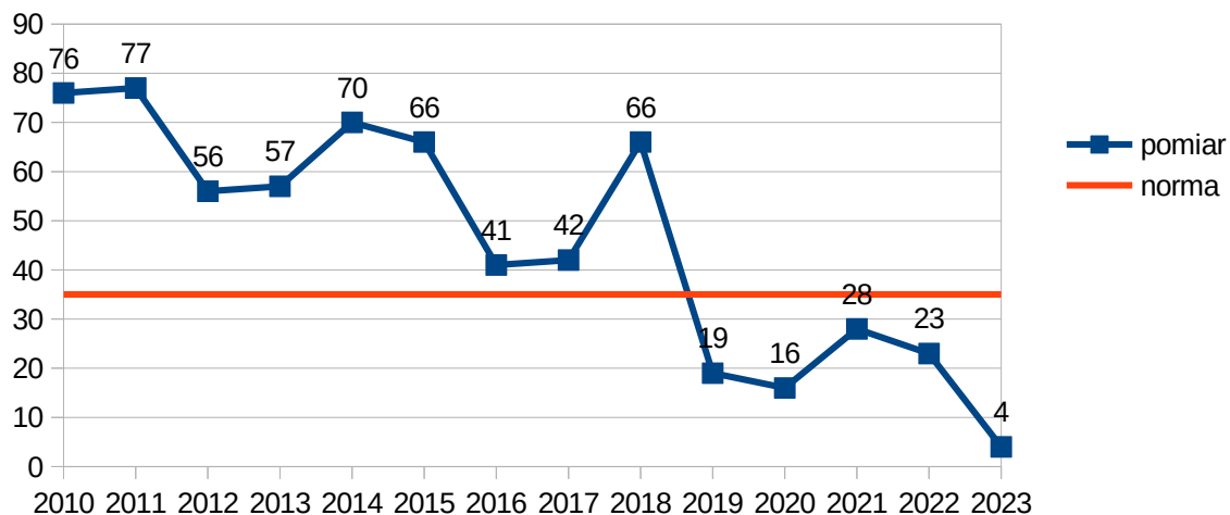
Wykres 9: Liczba dni w roku z przekroczonym dopuszczalnym stężeniem PM10. Opracowanie własne na podstawie danych WIOŚ.
